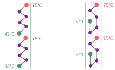
Нормальный конденсатор температура окр. среды 35°C e-pass форма прохода конденсатора температура окр. среды 35°C
